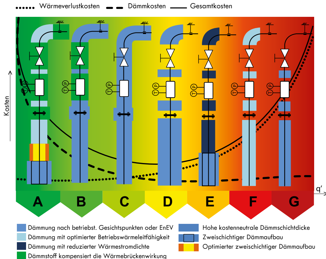
Grafik: Energieeffizienzklassen abhängig vom flächen- oder längenbezogenen Wärmeverluststrom, Auszug aus VDI 4610, Blatt 1, Grundriss
